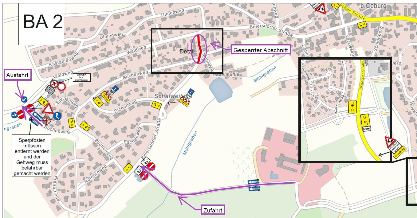
Verkehrszeichenplan Baustelle Beiersdorfer Straße, Quelle: CEB
